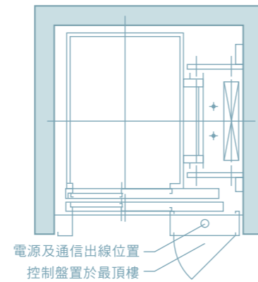
控制盤平面圖
