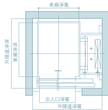
升降路平面圖
