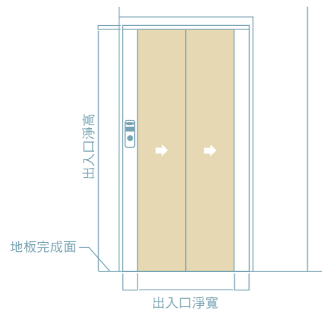
其它樓門框圖
