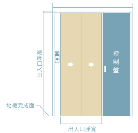
控制盤門框圖
