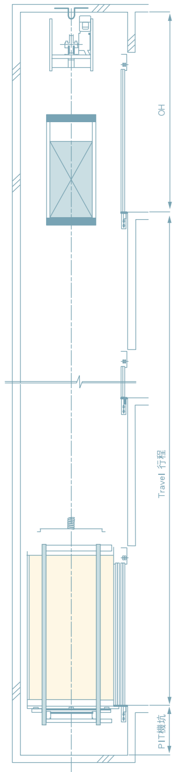
升降路剖面圖
